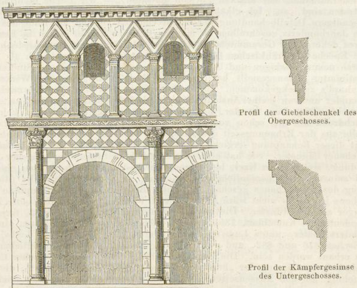
Von der Durchgangshalle zu Lorsch.
