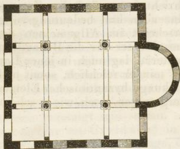
Dom zu Trier, ursprüngliche Anlage.
