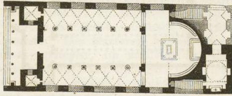
Grundriss von S. Croce in Gerusalemme zu Rom, vor der modernen Bauveränderung.
