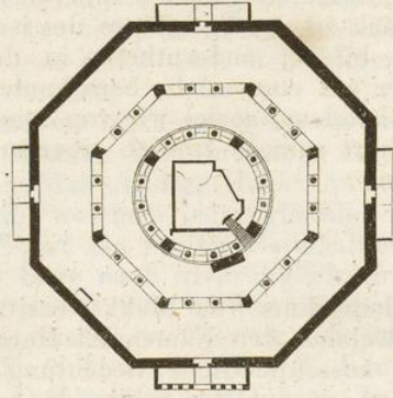
Grundriss der Moschee Omar's zu Jerusalem.
